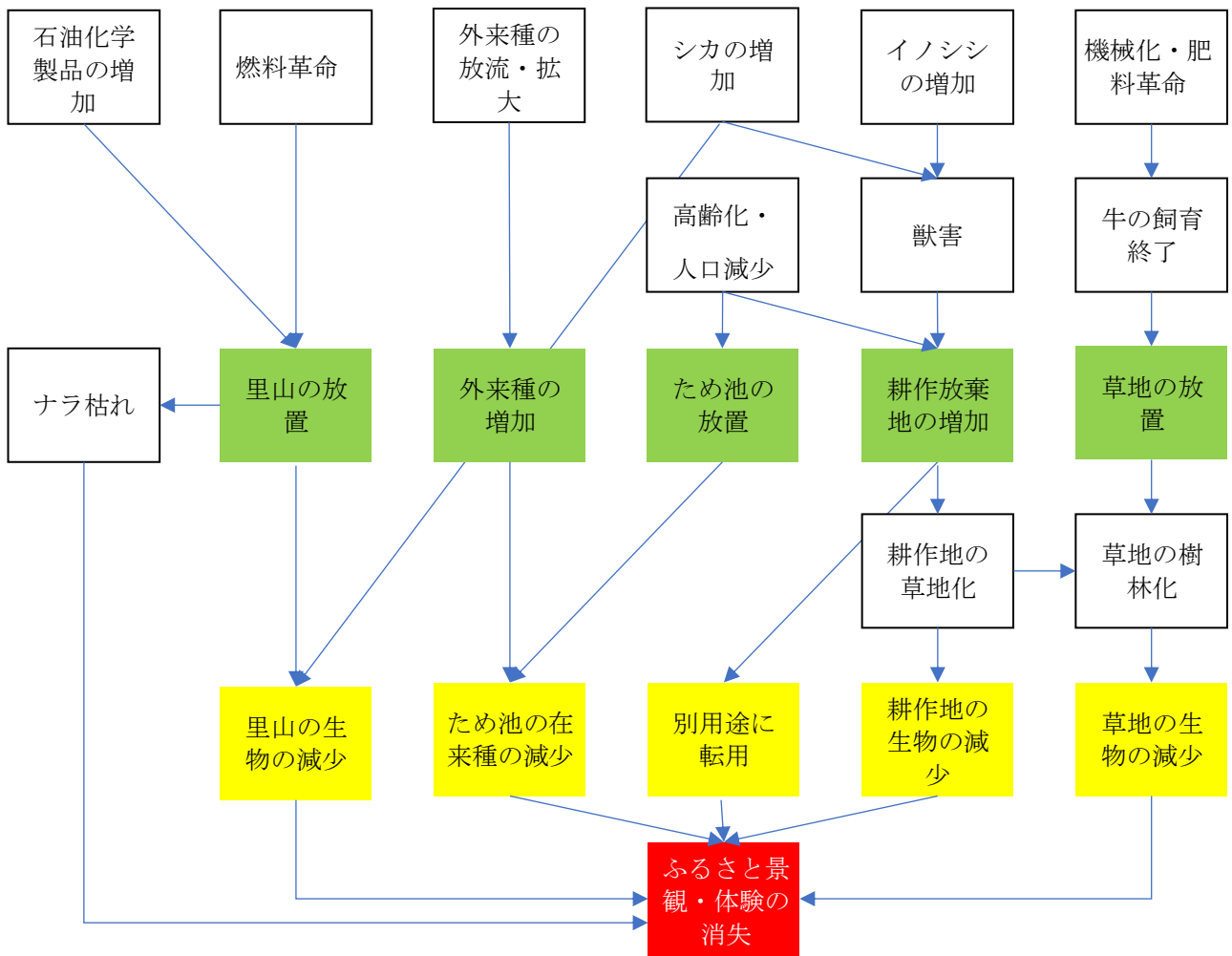
図1 ほしはら山のがっこう及び上田町の景観にかかわる相互関係 (緑：原因、黄：結果)
